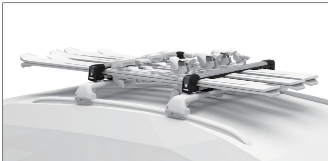
7322:W370mm×H110mm / バー上高さ:110mm(ローポジション時) / 139mm(ハイポジション時) 製品重量:2.8kg 7324:W620mm×H110mm / バー上高さ:110mm(ローポジション時) / 139mm(ハイポジション時) 製品重量:3.8kg 7326:W870mm×H110mm / バー上高さ:110mm(ローポジション時) / 139mm(ハイポジション時) 製品重量:4.8kg
